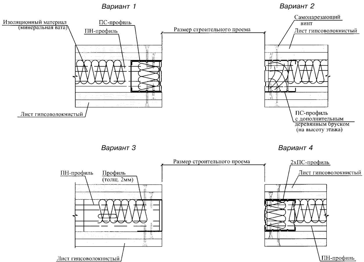
Рисунок 4 — Температурные швы и варианты дверных проемов в перегородках
