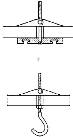
а - дюбель multifункциональный; б - дюбель для пустотелых конструкций; в и г - анкер проходной
