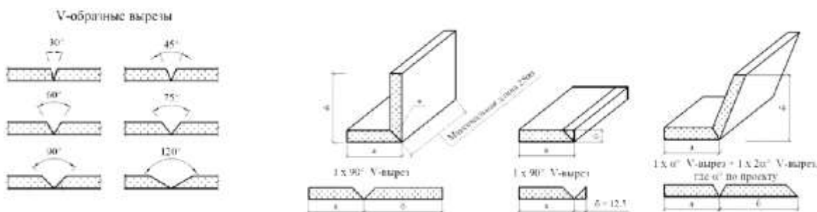
П-образные элементы конструкций ( a + b + v \leq 500 мм)
