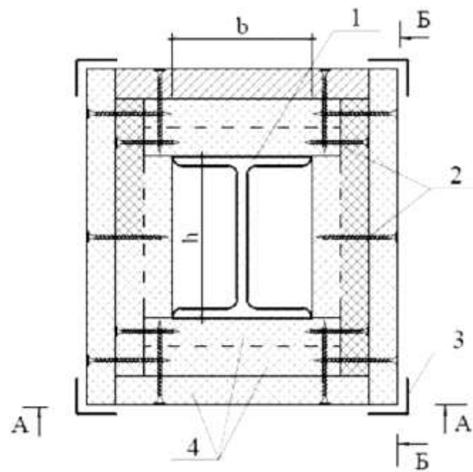
Вертикальные разрезы
