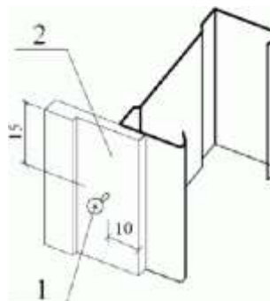
а - общий вид; б - крепление листов к стойке каркаса 1 - самонарезающий винт; 2 - лист ГКЛ или ГВЛ
