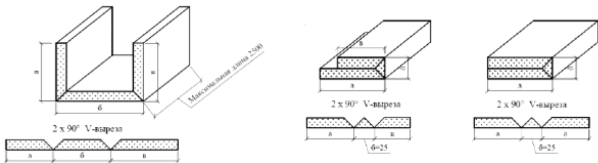
П-образные элементы конструкций ( a + b + c + h \leq 500 мм)
